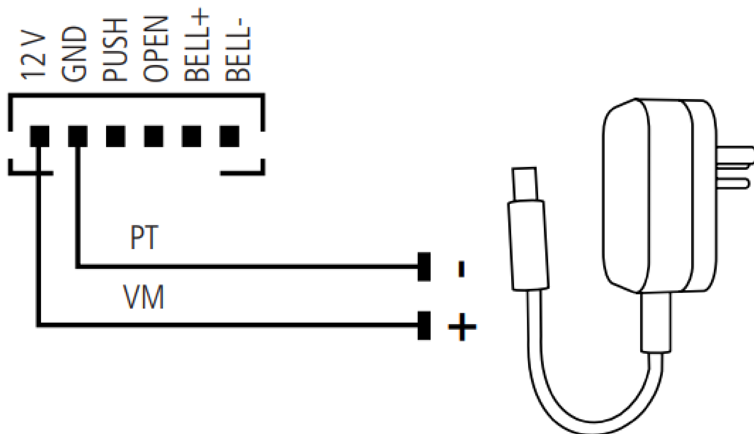
Fonte de alimentação
