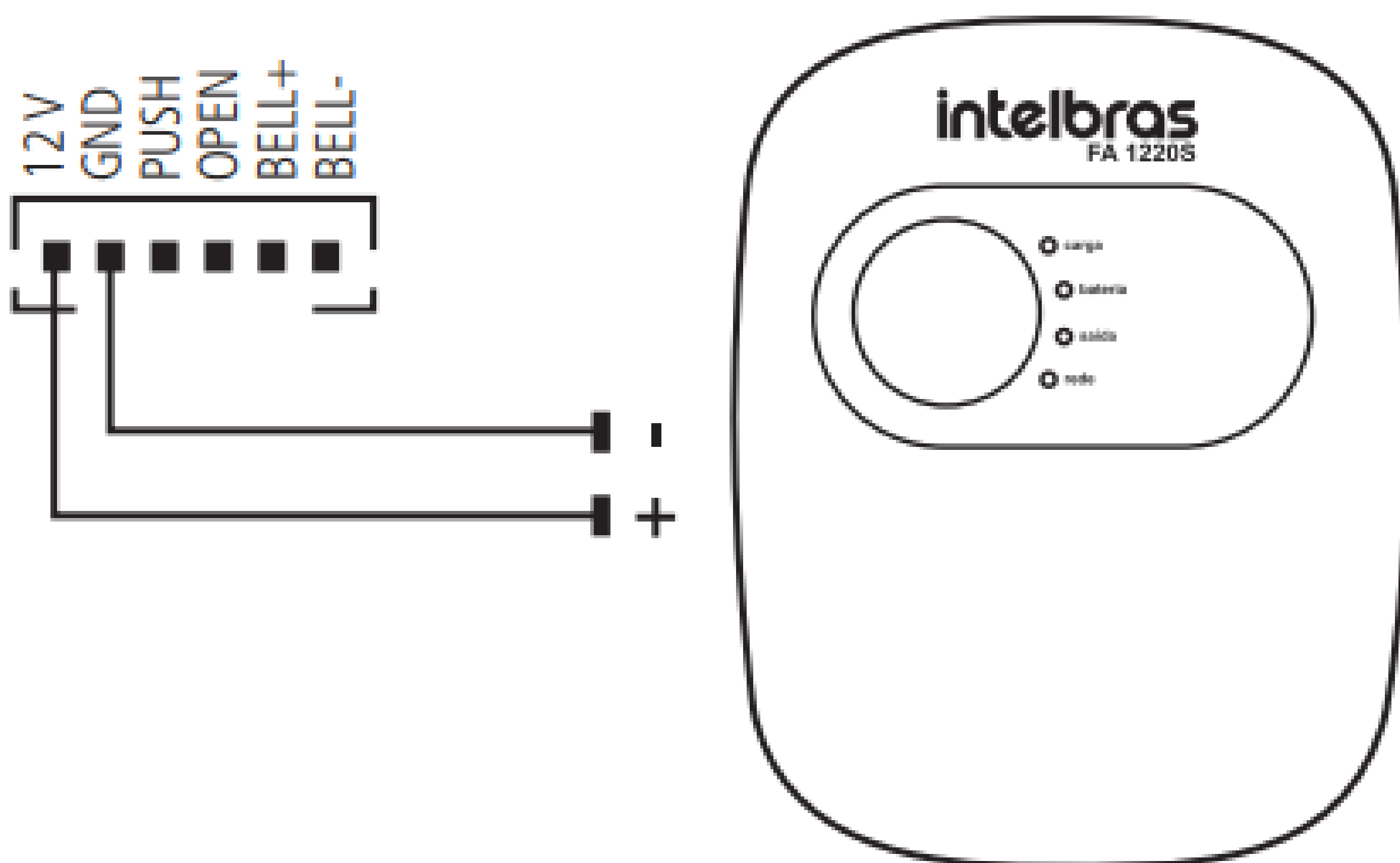
Fonte de alimentação com bateria
